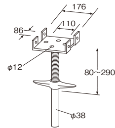
主要部材
