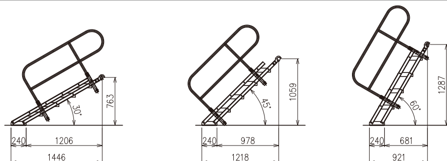
QS-15 設置例
