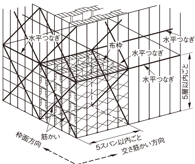
枠組支保工の連携
