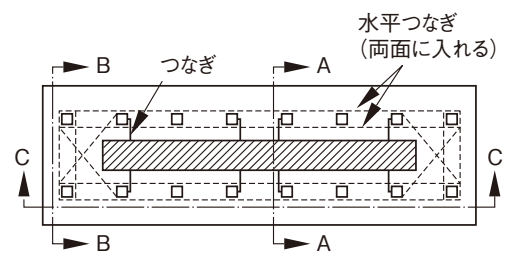
平面図②
