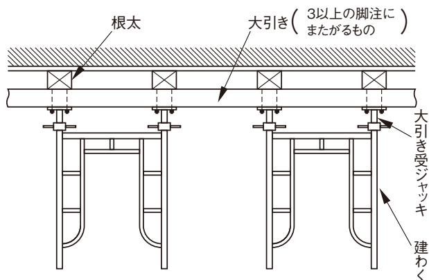
枠組支保工の連携
