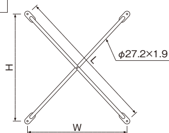
X プレース
