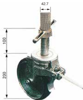
車輪 BL-8 (許容荷重: 1.96kN (200kg) : 1 ヶ)
