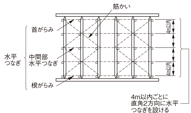
水平つなぎの間隔
