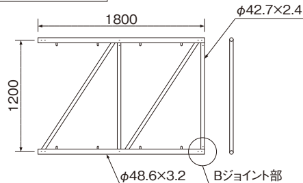
フレーム B-1218
