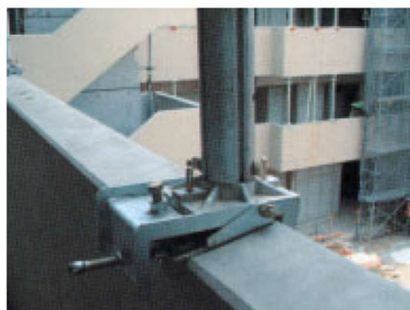
PCベース取付例
